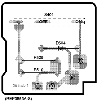
G STYLUS ILLUMINATOR SWITCH P.C.B.
