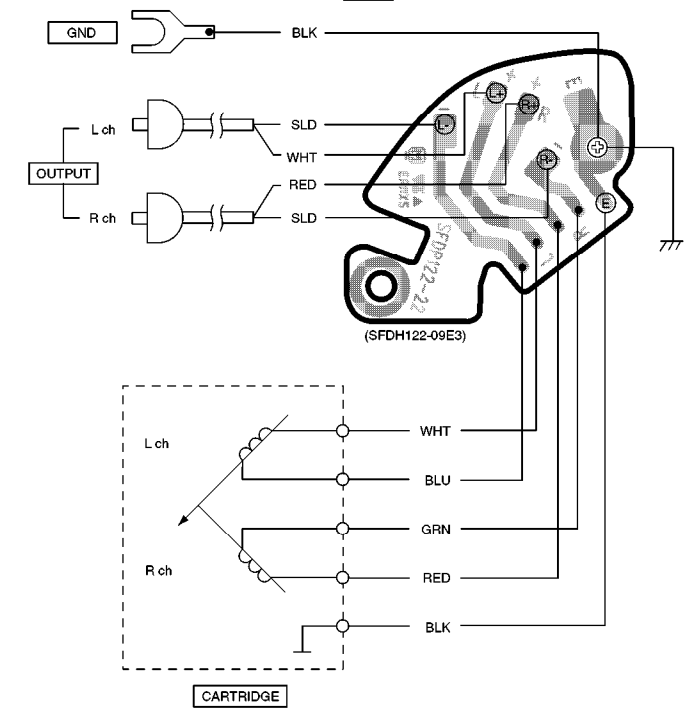
I OUTPUT P.C.B.
